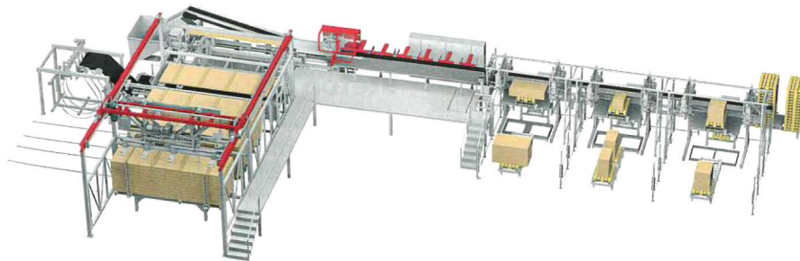
Vollautomatische Kappanlage mit Vakuumentapelung und Stapelmaschine (Reinhardt)
