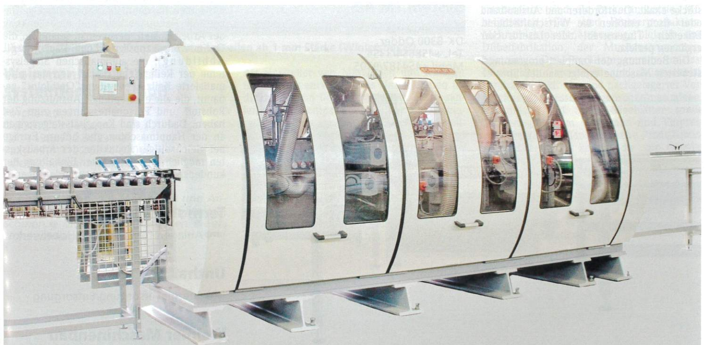
Längsprofiliermaschine „Duo 12 F“ für Fertigparkett (Schroeder)
