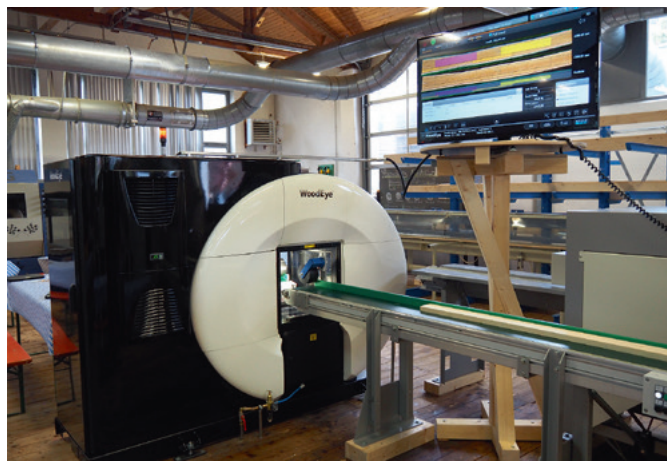
WoodEye stellte einen Scanner samt zweitem Bildschirm zur Verfügung – dieser ist drehbar, damit die Optimierung an der Kappsäge ersichtlicher ist
