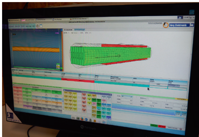
Genauere Darstellung: Die Jörg-Optimierung legt das Schnittbild aufgrund der hinterlegten Dimensionen in den zuvor gemessenen Stamm hinein
