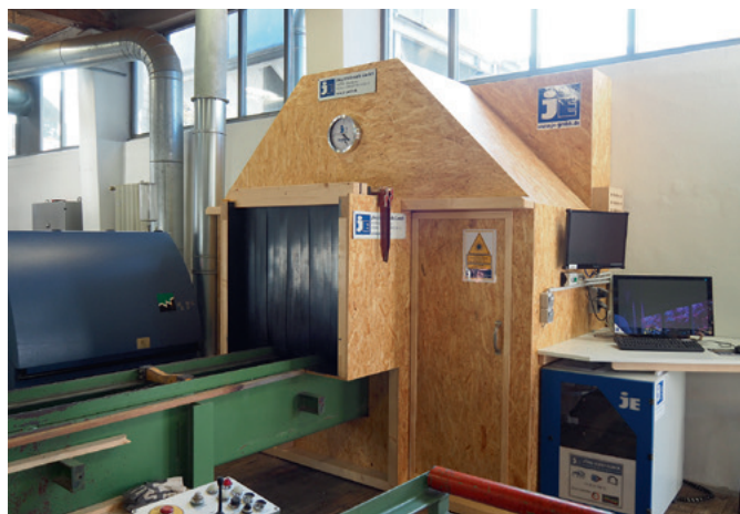
Rundholz-Messung von Jörg Elektronik: In dieser Umhausung befindet sich die Laser-Kamera-Technik
